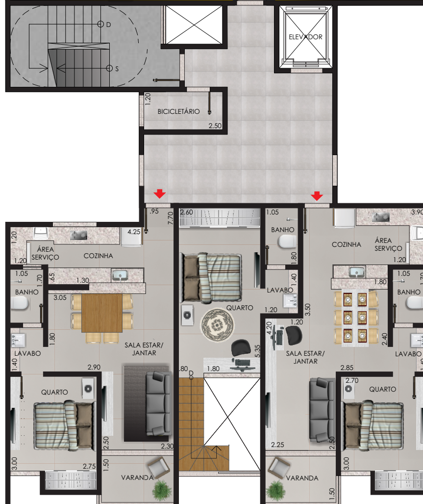
PLANTA BAIXA 5º, 7º e 9º PAVS - APTS TIPO
