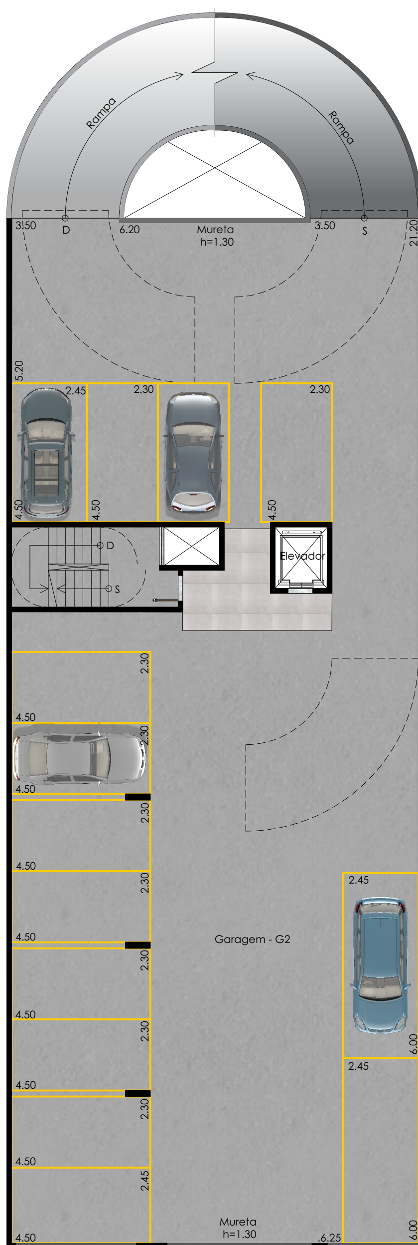
PLANTA BAIXA G2 - TORRE 01
